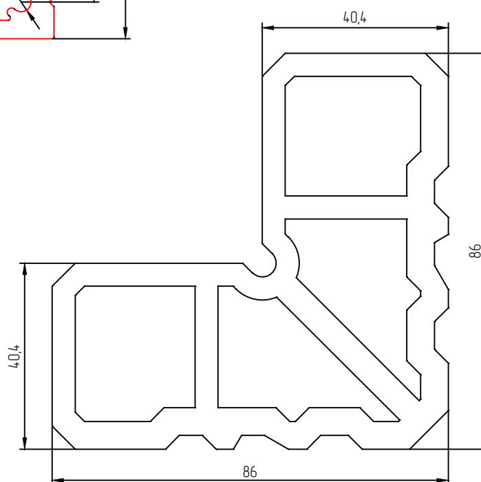
Сухарь угловой Код 10-713
