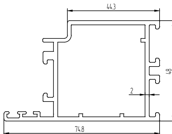
Рама двери внутреннего открывания Код 10-905
