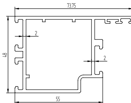
Рама двери наружного открывания Код 10-904
