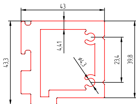
Сухарь импостный Код 10-931
