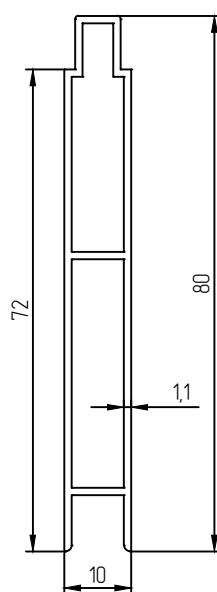
Ламбри двойной Код 130-102
