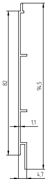
Ламбри одинарный Код 130-101
