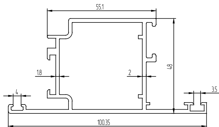
Створка двери наружного открывания Код 10-906
