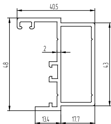
Адаптер низа двери Код 10-908
