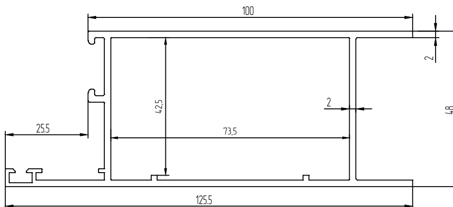
Низ двери Код 10-903
