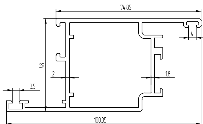
Створка двери внутреннего открывания Код 10-907
